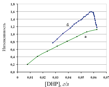
Рис. 4. Интенсивность поглощения DHP в ДМСО при разбавлении раствора большими (а) и маленькими (б) порциями.
