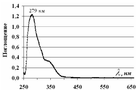
Рис. 3. УФ-спектр DHP в ДМСО с концентрацией 0,0625 г/л.
