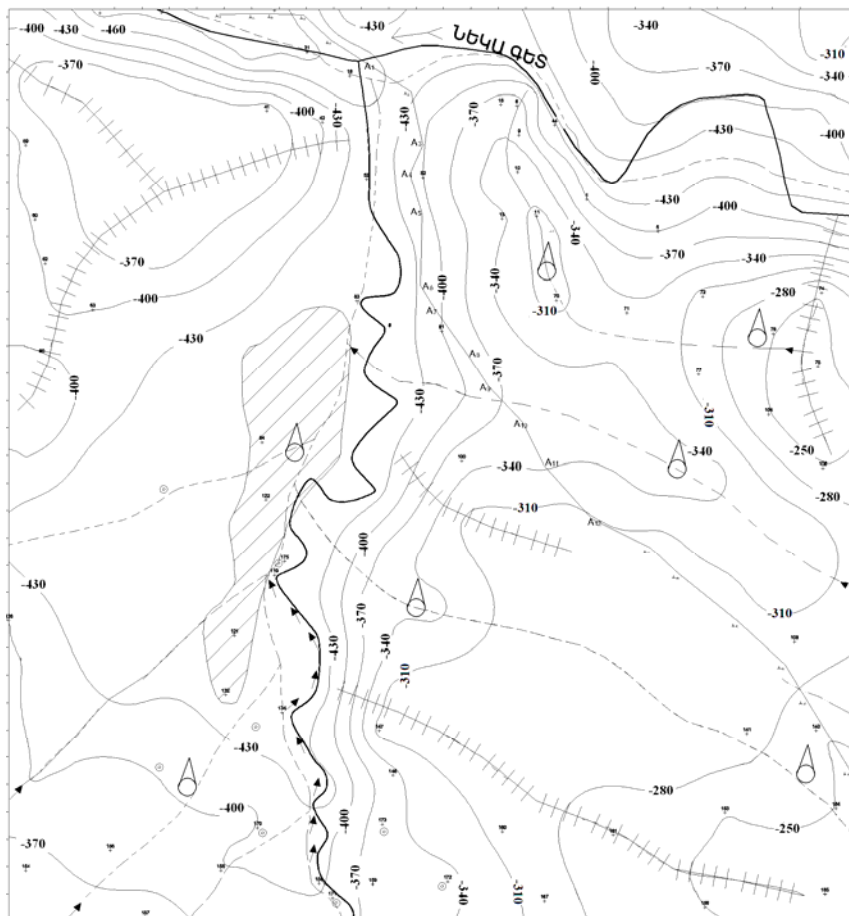
Նեկա գետի ջրհավաք ավազանի ջրամերժ շերտի ռելիեֆի սխեմատիկ քարտեզը:
