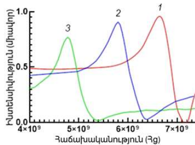
Նկար 9: Փոխանցման գործակիցների սպեկտրը S12 տարբեր երկարություններով ձողերի համար W=15 ; 17,5 ; 20 մմ, որոնք համապատասխանում են համապատասխանաբար 1,2,3 գրաֆիկներին: Այստեղ D=0.9\text{mm} , l=3\text{mm} , d=2\text{mm} :
