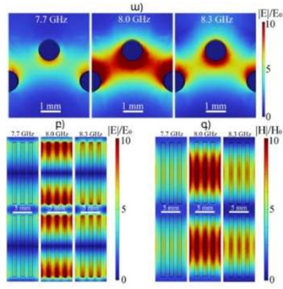
Նկար 4: Նորմալացված էլեկտրական դաշտի բաշխումը (ա) XY, (բ) XZ հարթություններում, և (գ) նորմալացված մագնիսական դաշտի բաշխումը XZ հարթությունում: Բաշխումները ներկայացված են ռեզոնանսային (8.0 ԳՀց) և \pm 300 ՄՀց տեղաշարժված հաճախականություններում: Բաժանարարի դիէլեկտրիկ թափանցելիությունը 1 է, իսկ երկրաչափական պարամետրերը նույնն են, ինչ Նկ. 3-ում: Սև եզրագծերը Cu-ի ձողերի սահմաններն են:
