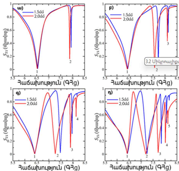
Նկար 13: TE 10 ուղղանկյուն ալիքատարի ռեժիմի չափված փոխանցման սպեկտրները, որոնք փոխազդում են փորձարկվող նմուշի հետ, որը բաղկացած է (ա) 2, (բ) 3, (գ) 4 և (դ) 5 պղնձե ձողերից բաղկացած գծային զանգվածից: Կապույտ գծերը համապատասխանում են ձողերի միջև 1.5 մմ հեռավորությանը, իսկ կարմիր գծերը՝ 2 մմ հեռավորությանը:
