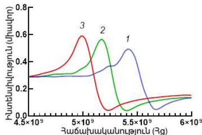
Նկար 10: S_{12} անցման գործակիցի սպեկտրները ձողի տրամագծերի փոփոխության դեպքում՝ D=0.6 ; 0.9 ; 1.1 մմ, որոնք համապատասխանում են համապատասխանաբար 1, 2, 3 գրաֆիկներին: Այստեղ W=20\text{մմ} , l=3\text{մմ} , d=2\text{մմ} :
