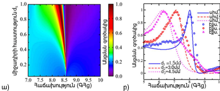
Նկար 5: ա) Փոխանցման ուղվագծային քարտեզը, որը ցույց է տալիս անցանելիությունը՝ կախված հաճախականությունից և միջադիրի հաստությունից, որն փոփոխվում է 0.05 մմ-ից մինչև 1 մմ: բ) Փորձարարական (նշաններով) և մոդելավորված (գծերով) անցանելիության սպեկտրները՝ տարբեր BMS միջադիրի հաստությունների համար: Մնացած բոլոր գեոմետրիկ պարամետրերը նույնն են, ինչ նկար 3-ում:
